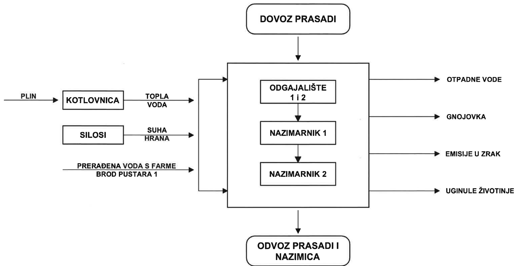
Prilog 2. Blok dijagram tehnološkog procesa na Farmi Brod Pustara 2
